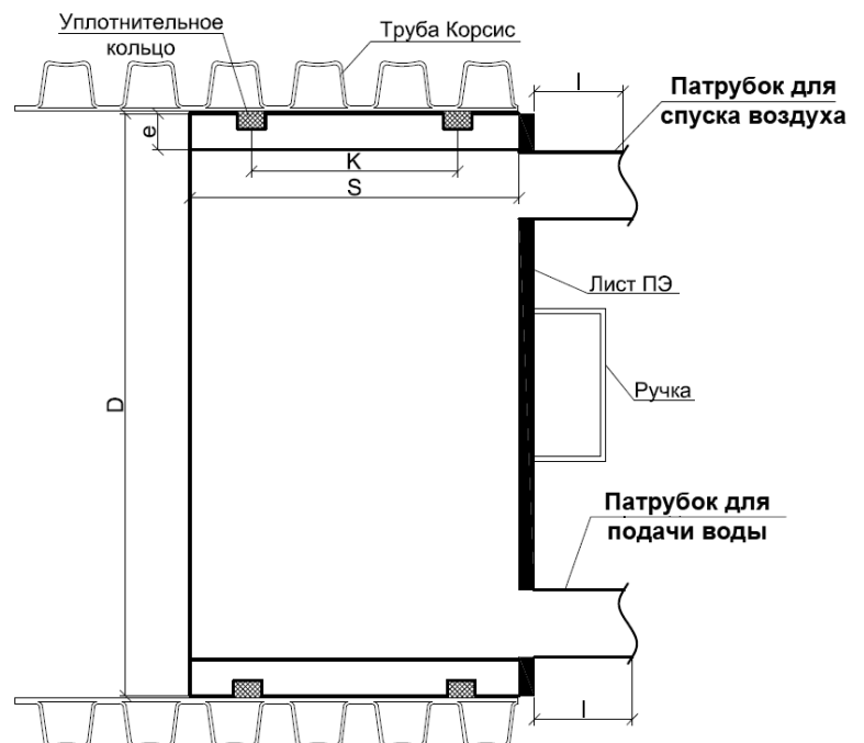
Рисунок 5. Заглушка внутренняя
